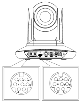
VISCA IN &Mini DIN Connection
